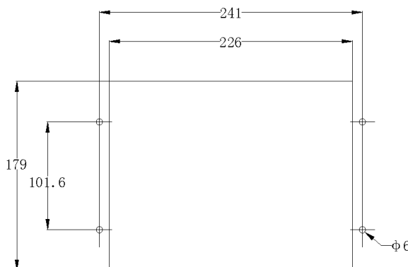
图 3-2 开孔尺寸
