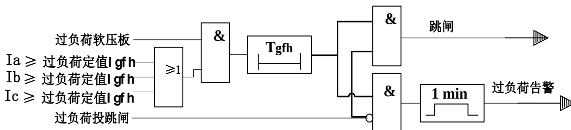
图 5-3 过负荷原理图
