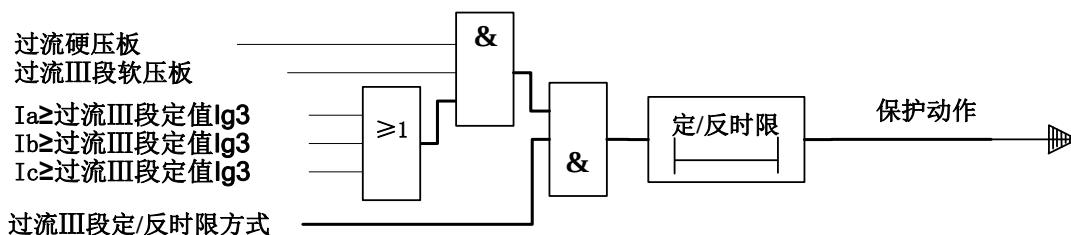
图 5-2 过流 III 段原理图
