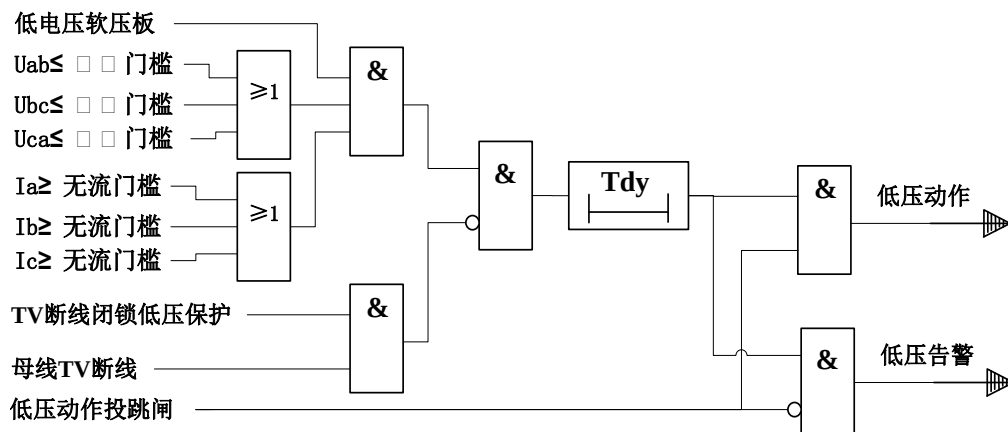
图 5-5 低电压保护原理框图
