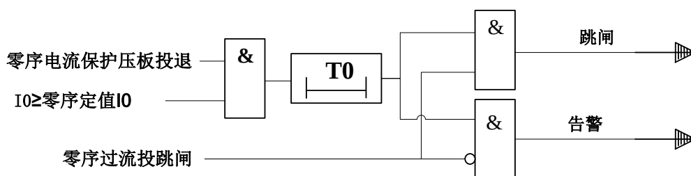
图 5-4 零序过流保护原理
