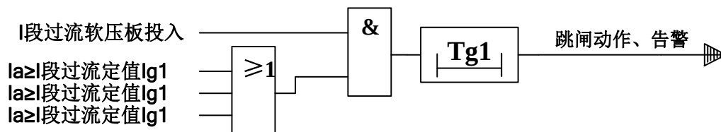
图 5-1 过流 I 段原理图
